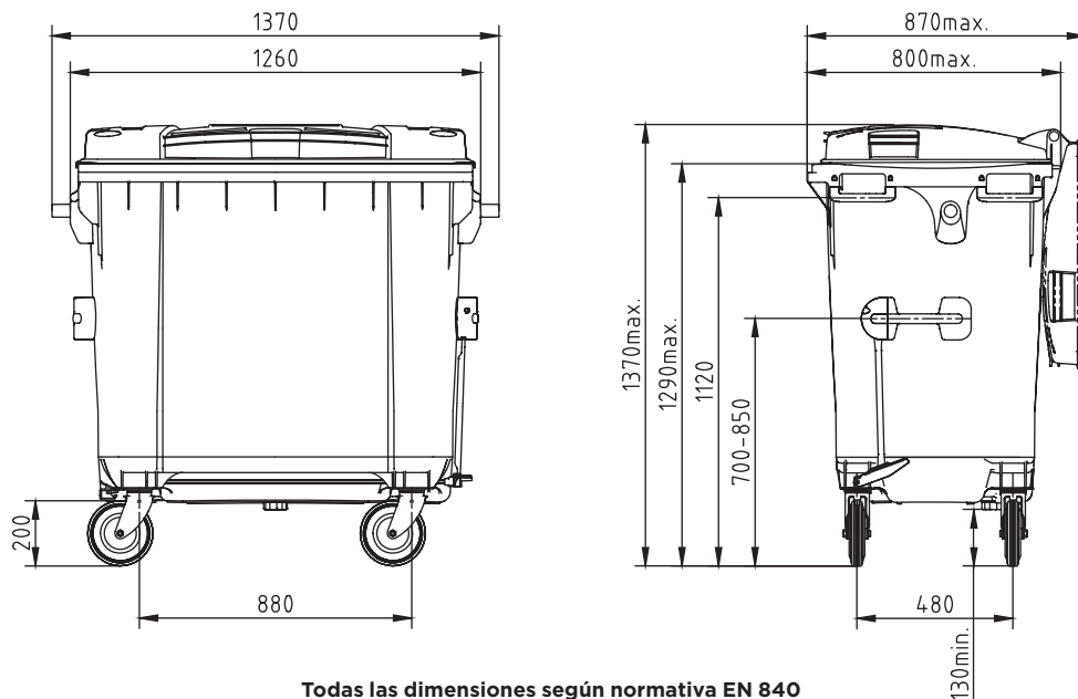
Todas las dimensiones según normativa EN 840
